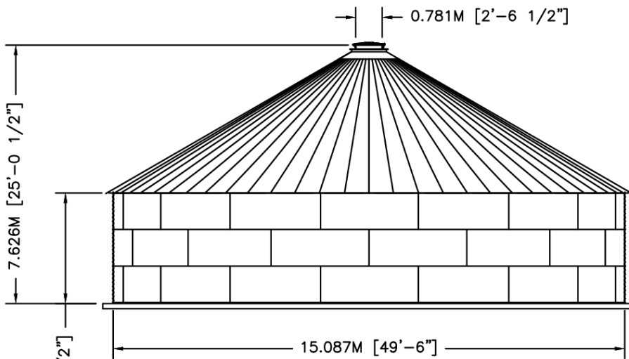
ELEVATION
